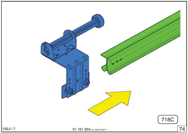
106J1-7 01 161 994 rev. 28-07-2017 74
