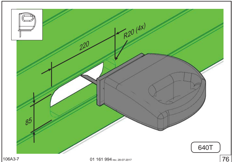
106A3-7 01 161 994 rev. 28-07-2017 76
