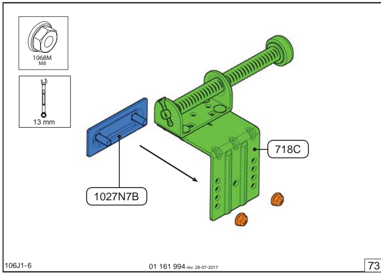
106J1-6 01 161 994 rev. 28-07-2017 73
