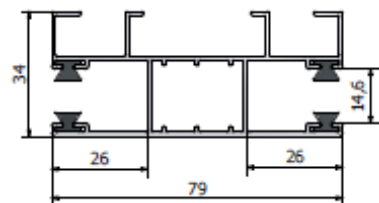
N/PPD79 stosowane z PPD79, PPD79/ODS + płytka PZO
