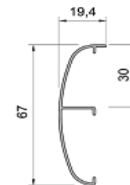
N/PP66 stosowane z PP66 + płytka PZO
