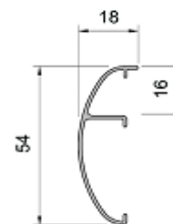
N/PPDO stosowane z PP53, PP53/ODS, PK53, PPDO53, PPMO53 + płytka PZO
