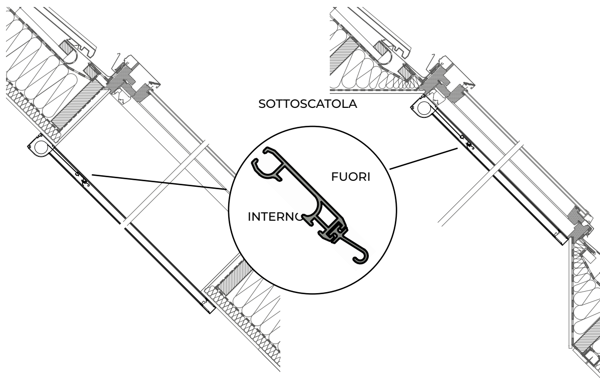
Zanzariera avvolgibile [lucernario, installazione all'esterno del vano]
