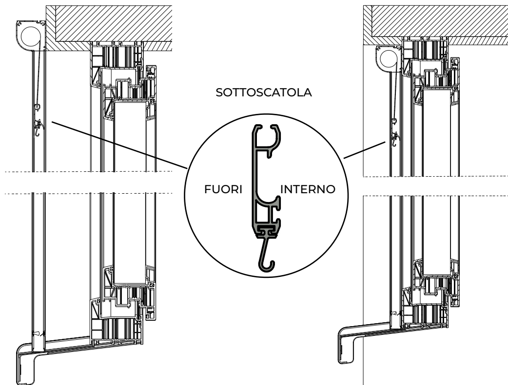
Zanzariera avvolgibile [finestra standard, installazione all'esterno del vano]
